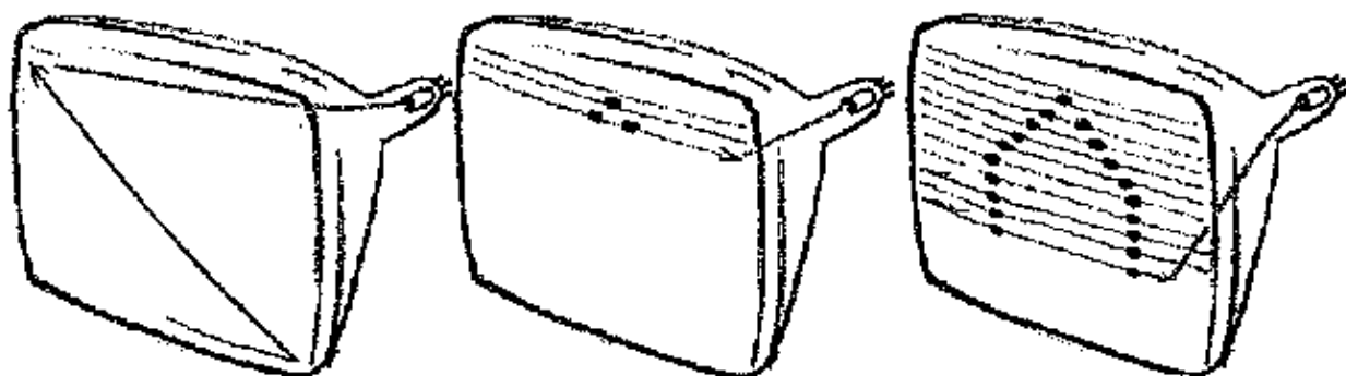
Рис. 4.9. Получение растрового изображения в электронно-лучевой трубке
