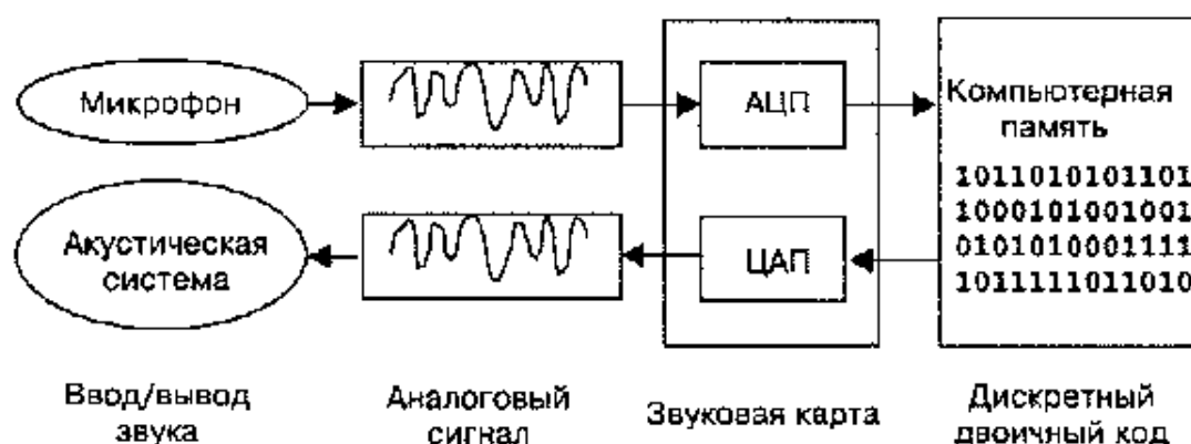
Рис. 5.3. Преобразование звука при вводе и выводе
