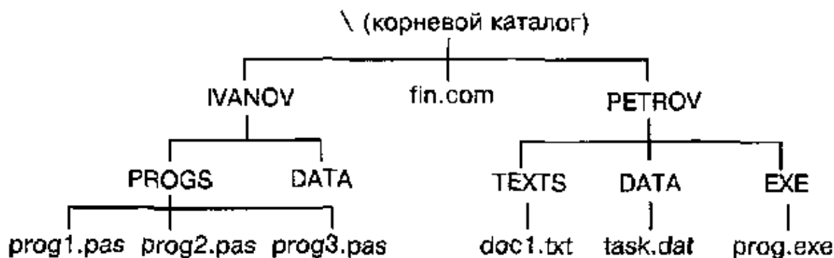
Рис. 2.9. Пример иерархической файловой структуры
